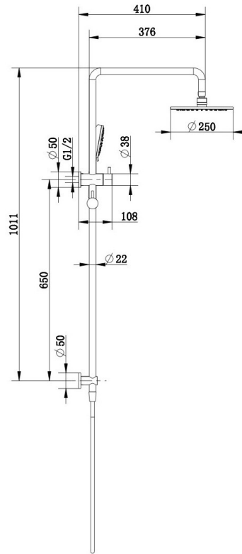
比例 1:10
